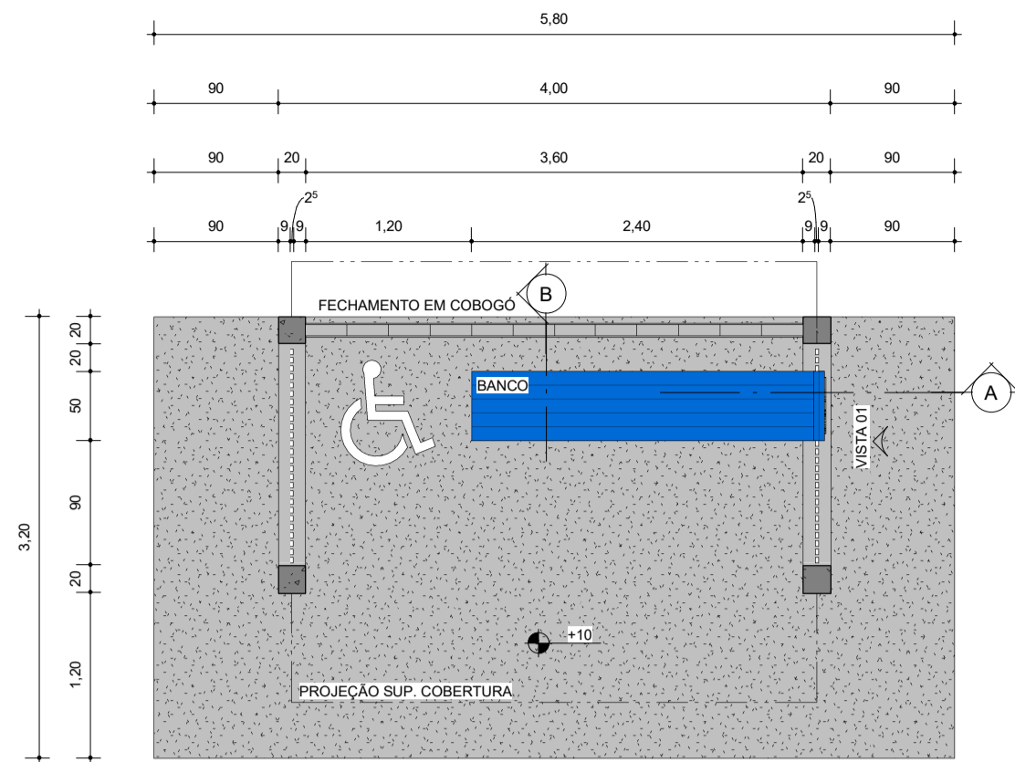
PLANTA BAIXA
