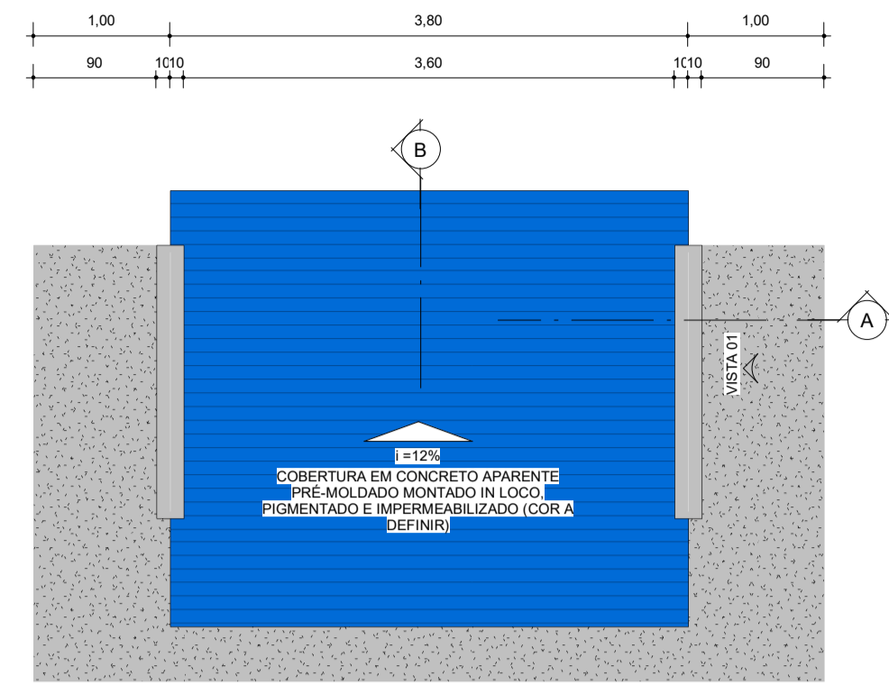
COBERTURA
