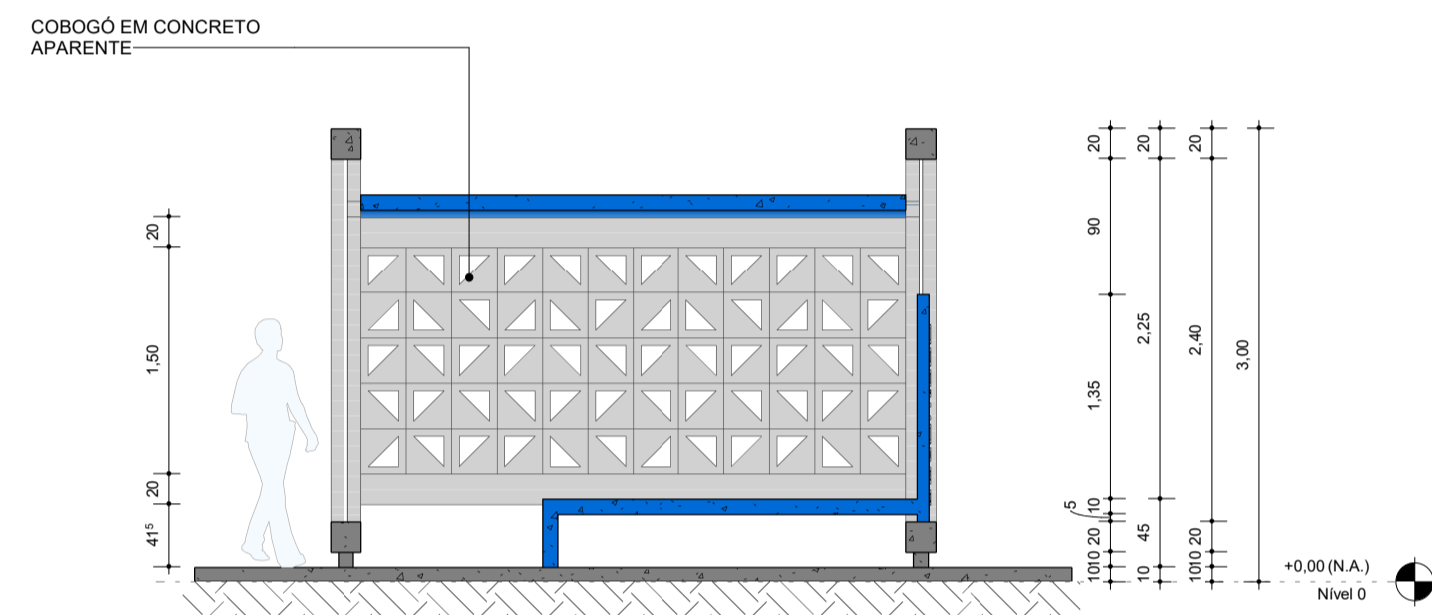
CORTE A
