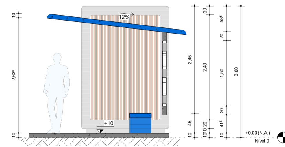
CORTE B
