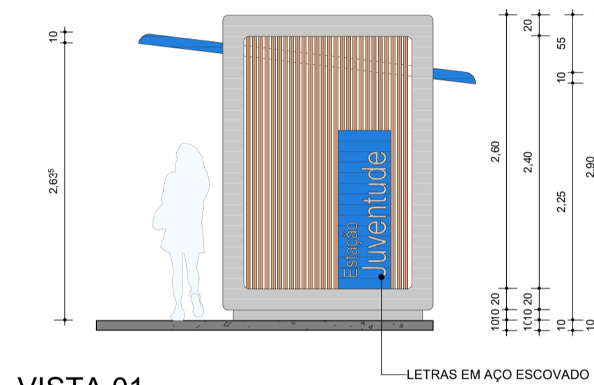
VISTA 01
